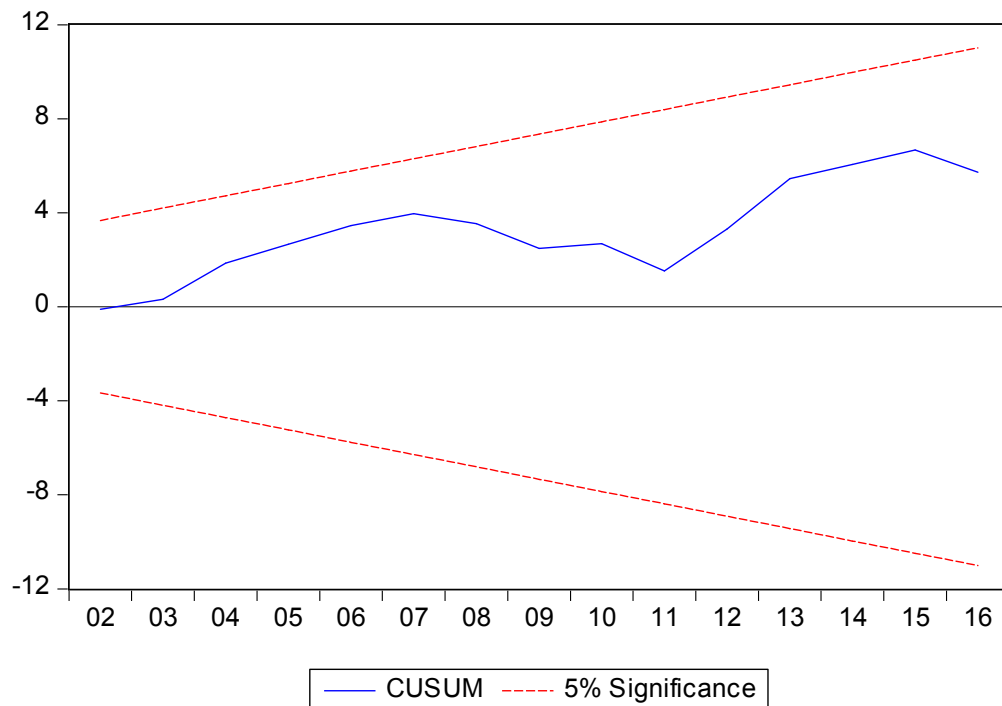
Fig. 3. CUSUM test
